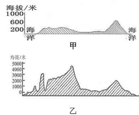
图 16 地形剖面图
